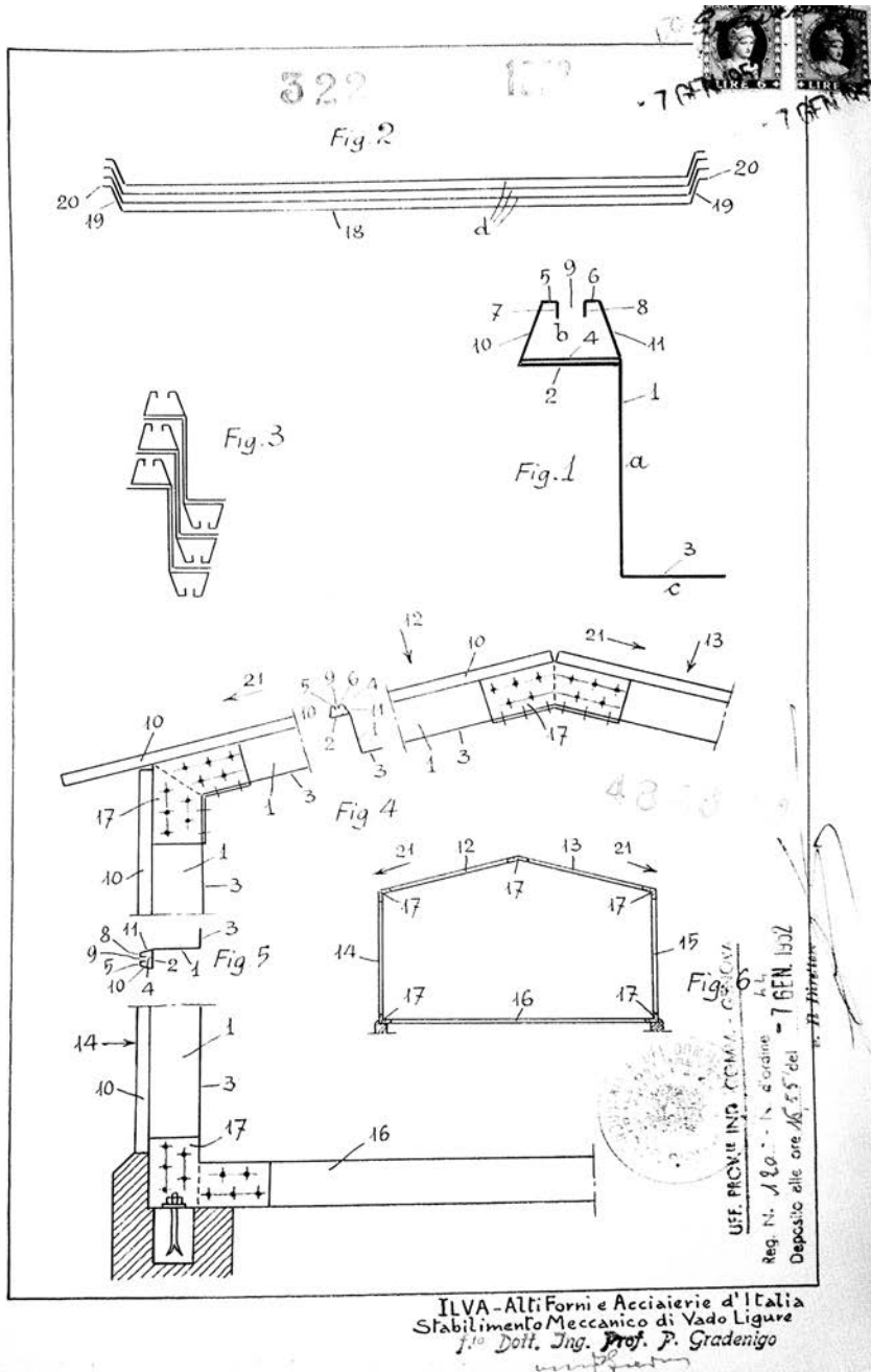
Fig. 11 – ILVA, brevetto n. 484674, “Padiglione smontabile in elementi metallici e lamine o lamiere nonché elementi metallici a sezione particolare”, depositato il 7 gennaio 1952 (ACS, UIBM).
