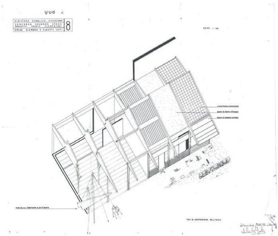
Fig. 7 – Concorso per scuole elementari di campagna e montagna, proposta di Alberto Gatti e Diambra de Sanctis, assonometria del montaggio, 1952 (AMPI, DGES, Fondo ESS)
