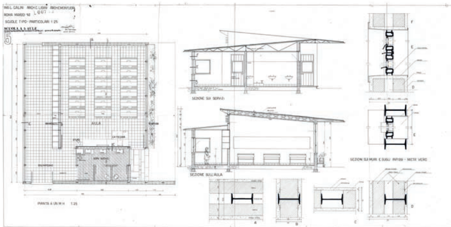
Fig. 10 – Concorso per scuole elementari di campagna e montagna, proposta di Leo Calini, Cesare Ligini, Eugenio Montuori, assonometria della struttura metallica prodotta dalla Società ILVA, sezioni con dettagli della struttura e degli infissi in ferro finestra, 1952 (AMPI, DGES, Fondo ESS)
